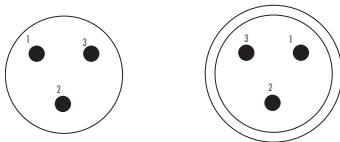
Gehäuse 2 12 x ø 1,6 mm
