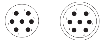
Gehäuse 1 4 x ø 2,4 mm
