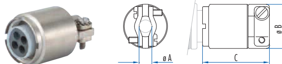
Kabelklemme für Natto Miniatur Push-Pull
