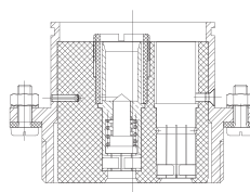
Gerätesteckverbinder
