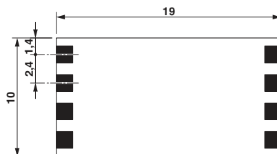
Maßzeichnung
